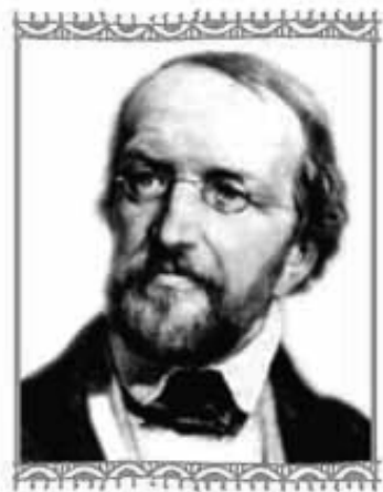
Lejeune Dirichlet (1805-1859)
