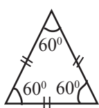
समबाहु त्रिभुज
