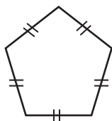
सम पंचभुज
