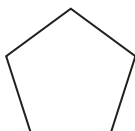
पंचभुज
